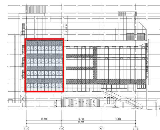
公園側立面図
