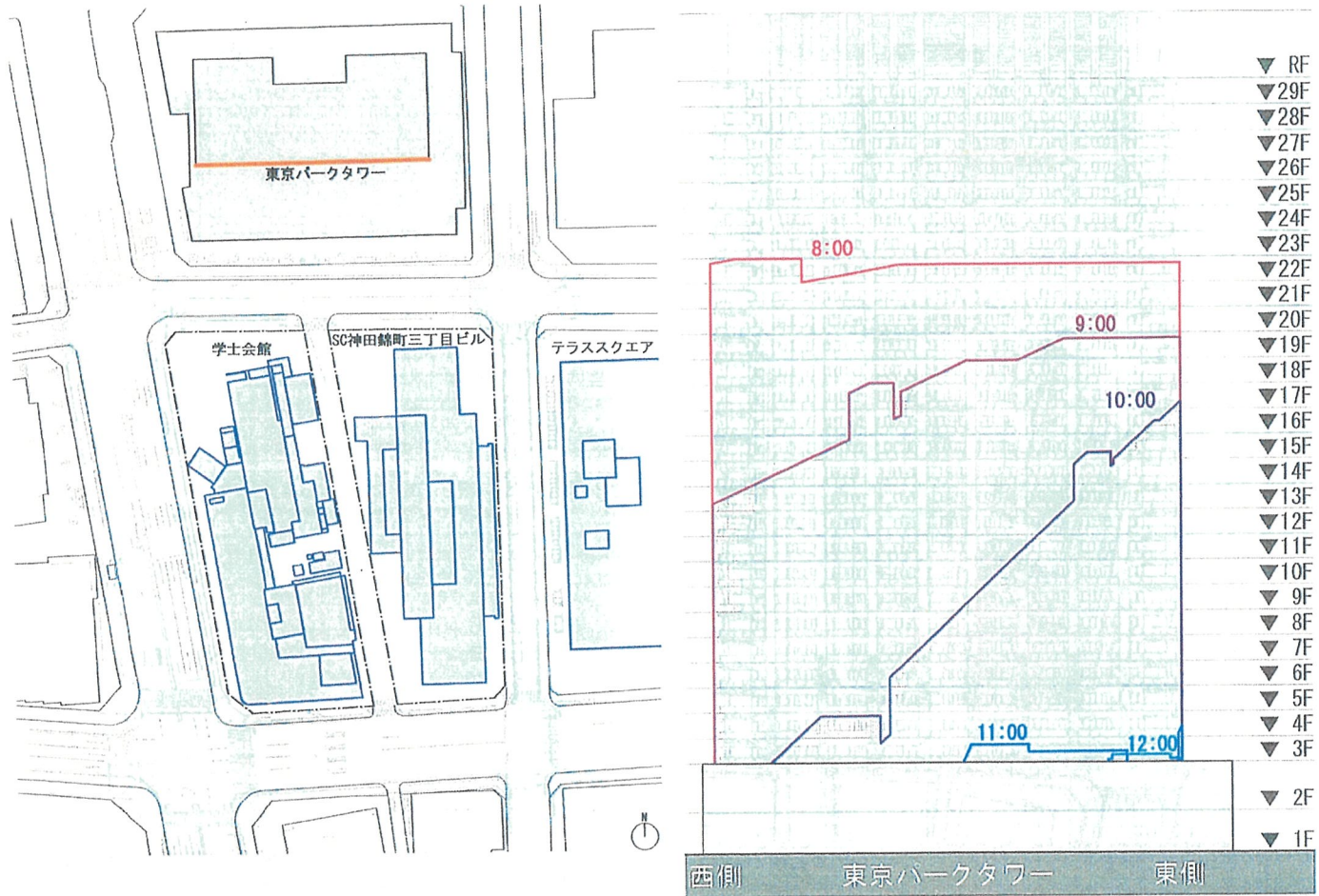
壁面時刻日影図 冬至
